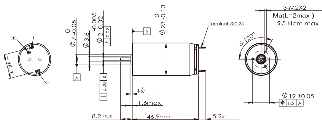
电机参数 Motor Data
