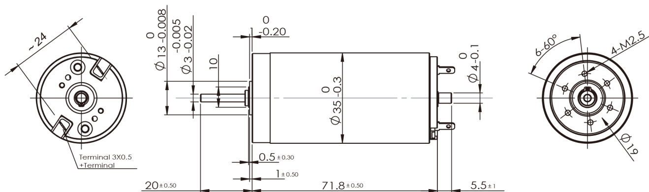
电机参数 Motor Data
