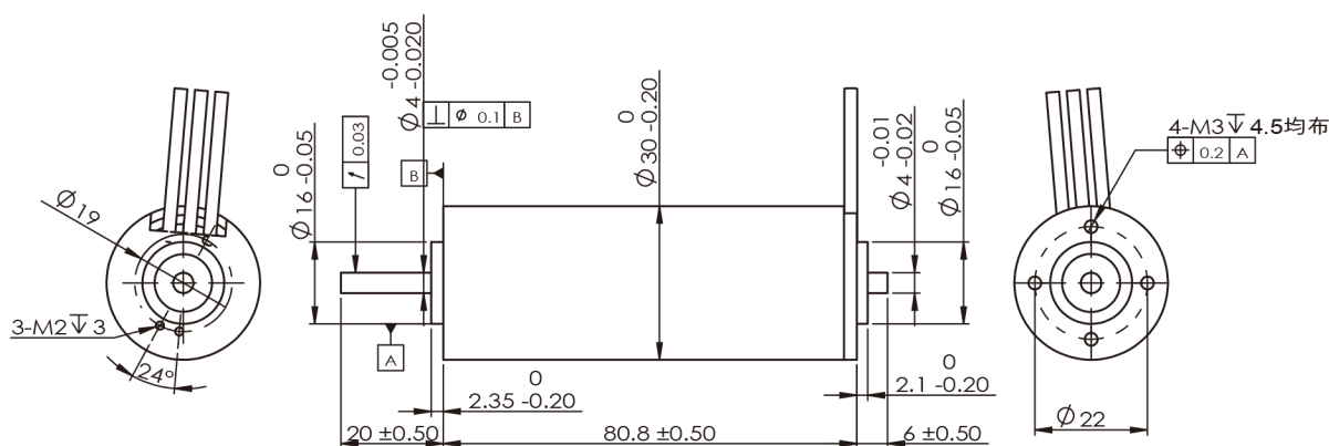
电机参数 Motor Data
