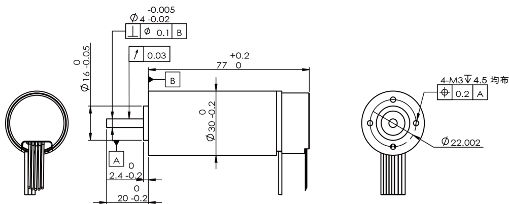
电机参数 Motor Data
